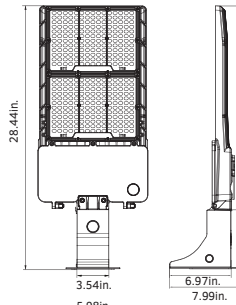
250W / 300W (Wall Mount)
